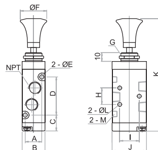
Válvulas 5/2
