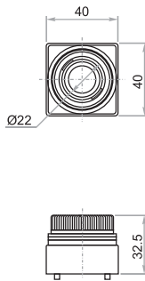
BS - Botón Rasante
