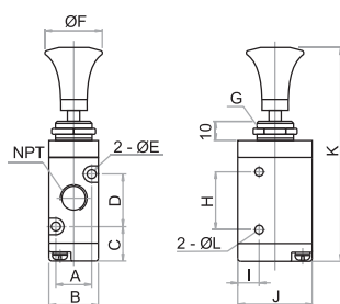
Válvulas 3/2
